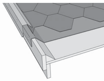
Kerabit Takgavelplåt för trekantslist
